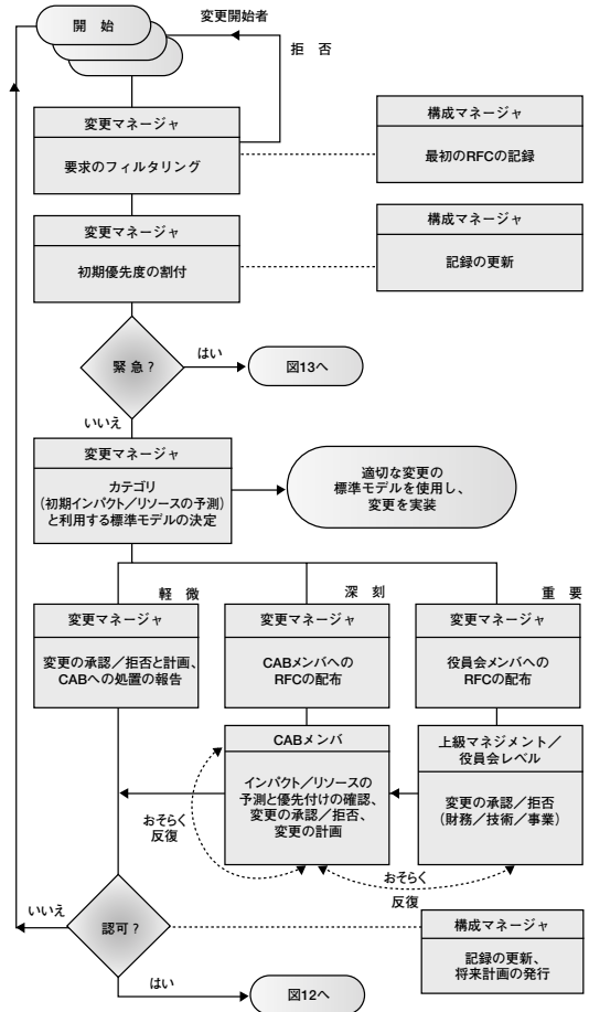
図11：変更手順 - パート1 (通常の場合)
